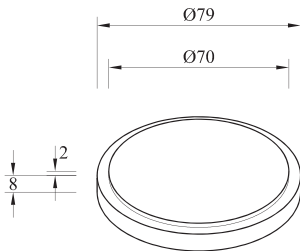
P2RH.36 Blanking Cap Trespa® HPL
